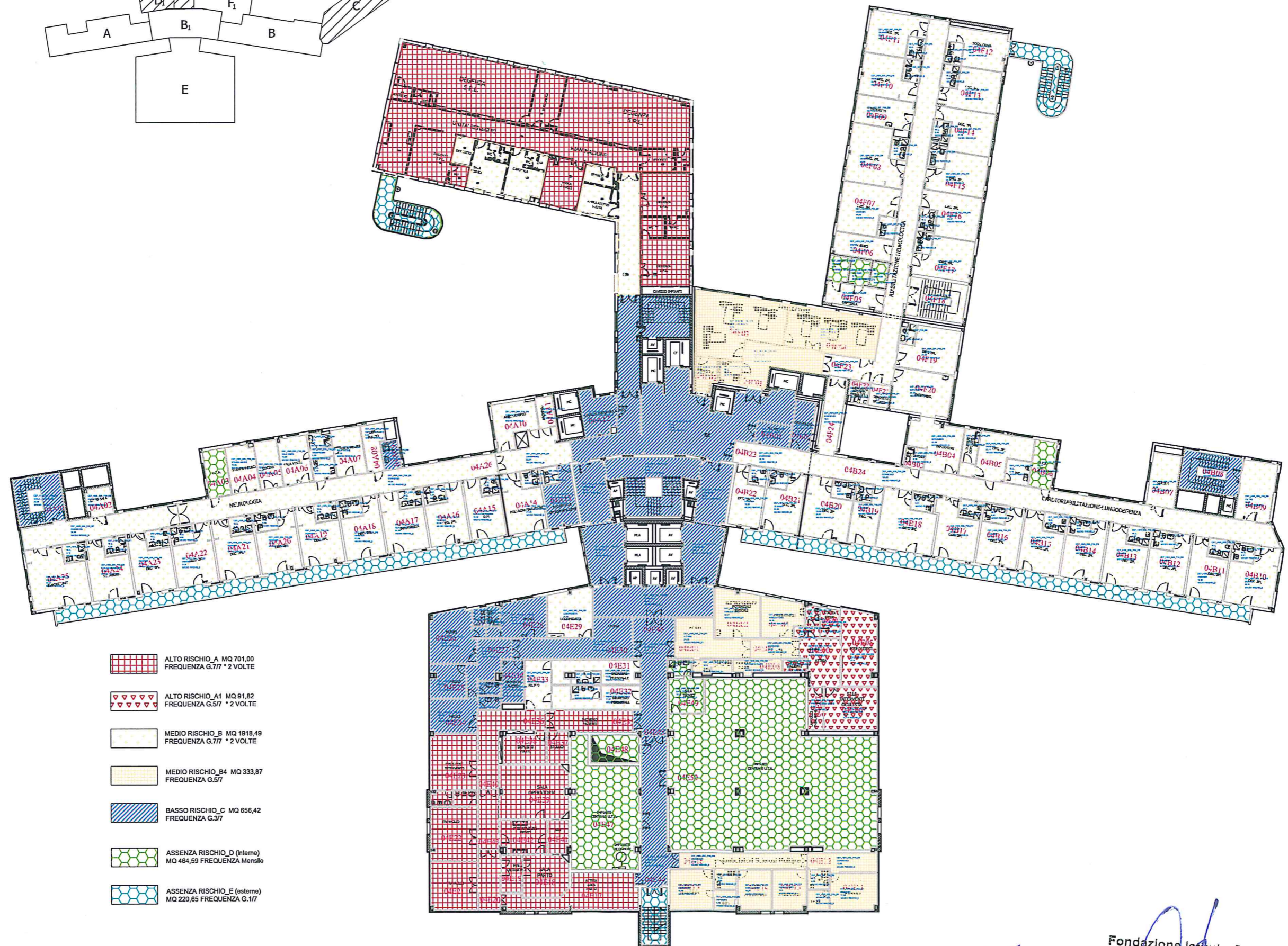
PIANTA PIANO QUARTO
